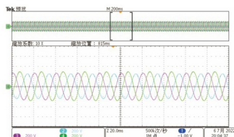
IEC61000-4-27 电压不平衡@Class3
