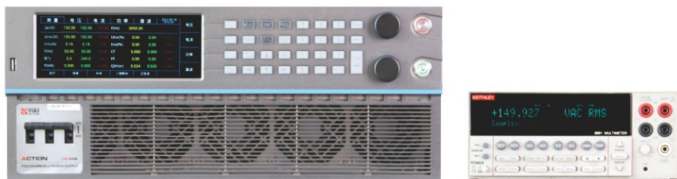
PRE15输出150V实测电压精度：0.016% F.S.
