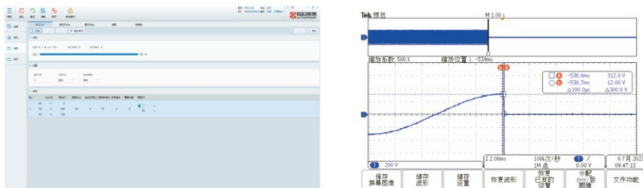
基波：AC220V/50Hz 90° 电压跌落，跌落时间 100\mu\text{s}@90\%\sim 10\%
