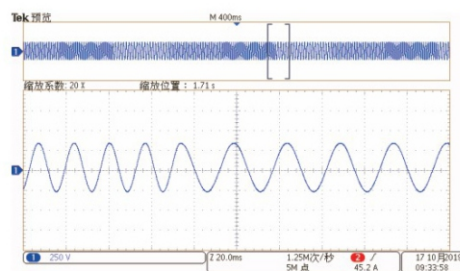
IEC61000-4-28 工频变化@Class4
